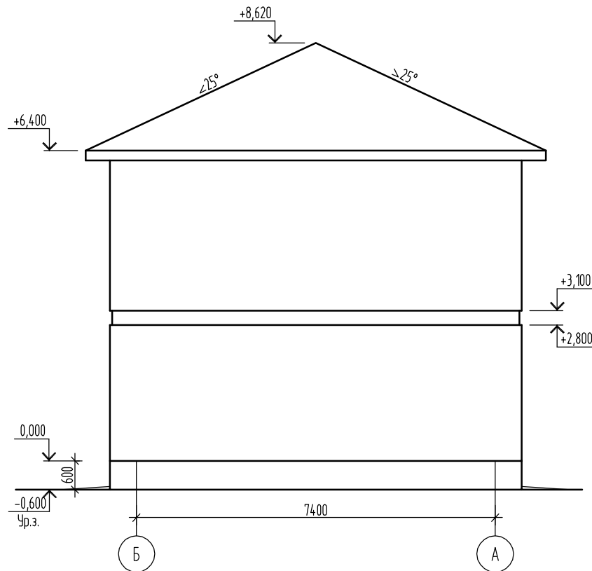
Фасад Б-А
