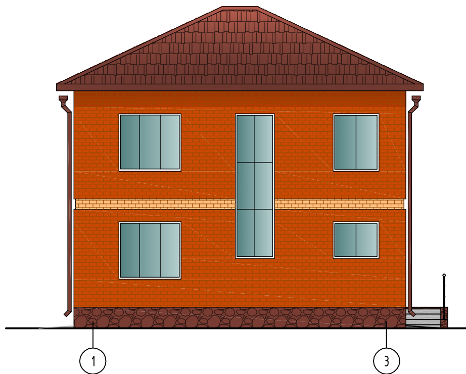
Фасад 1-3
