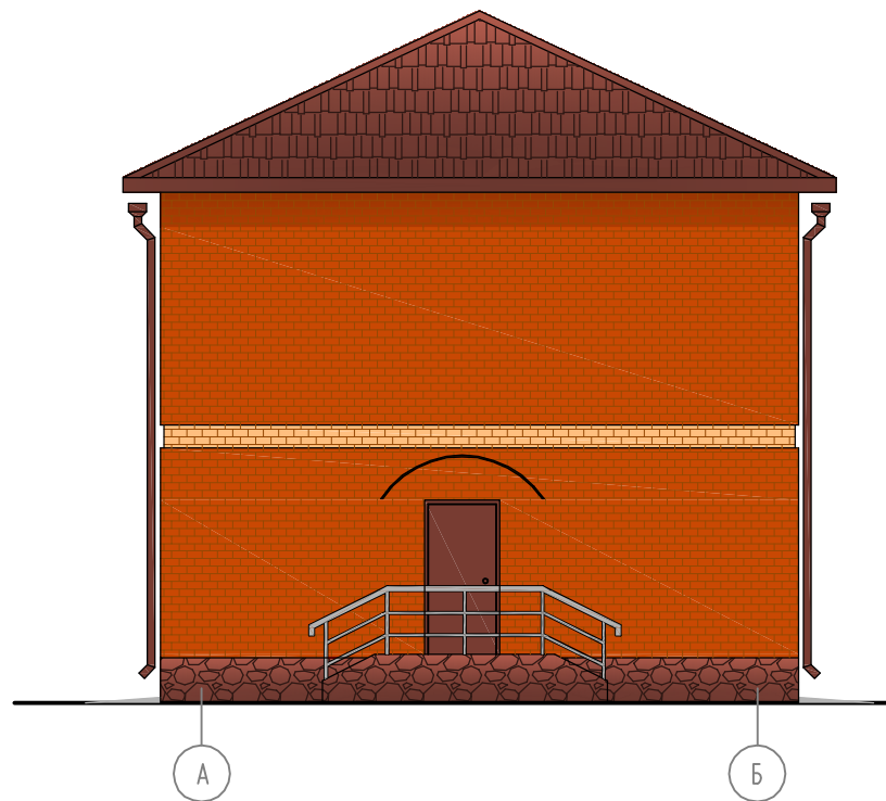
Фасад А–Б
