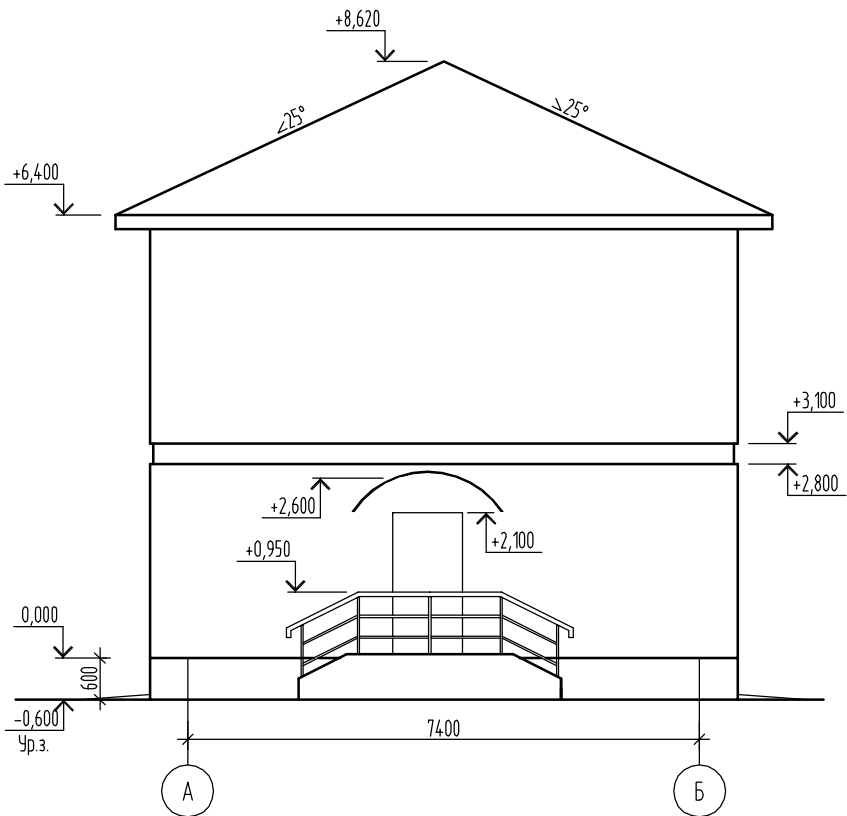
Фасад А-Б
