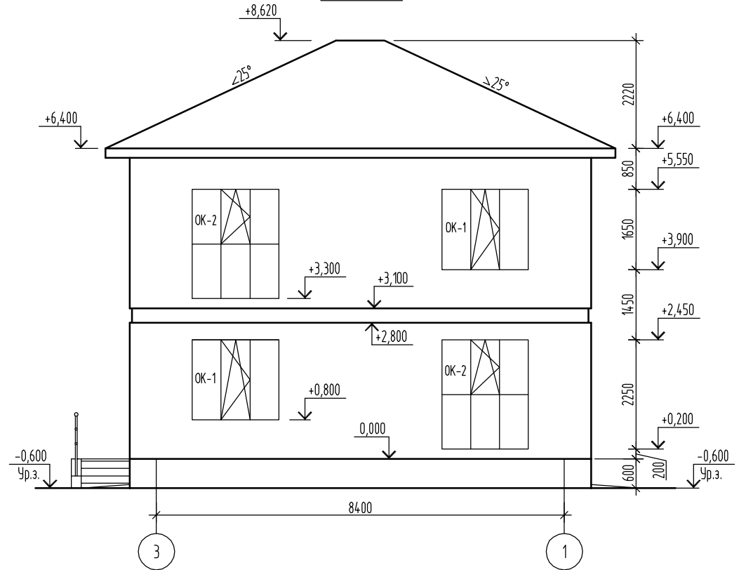
Фасад 3-1
