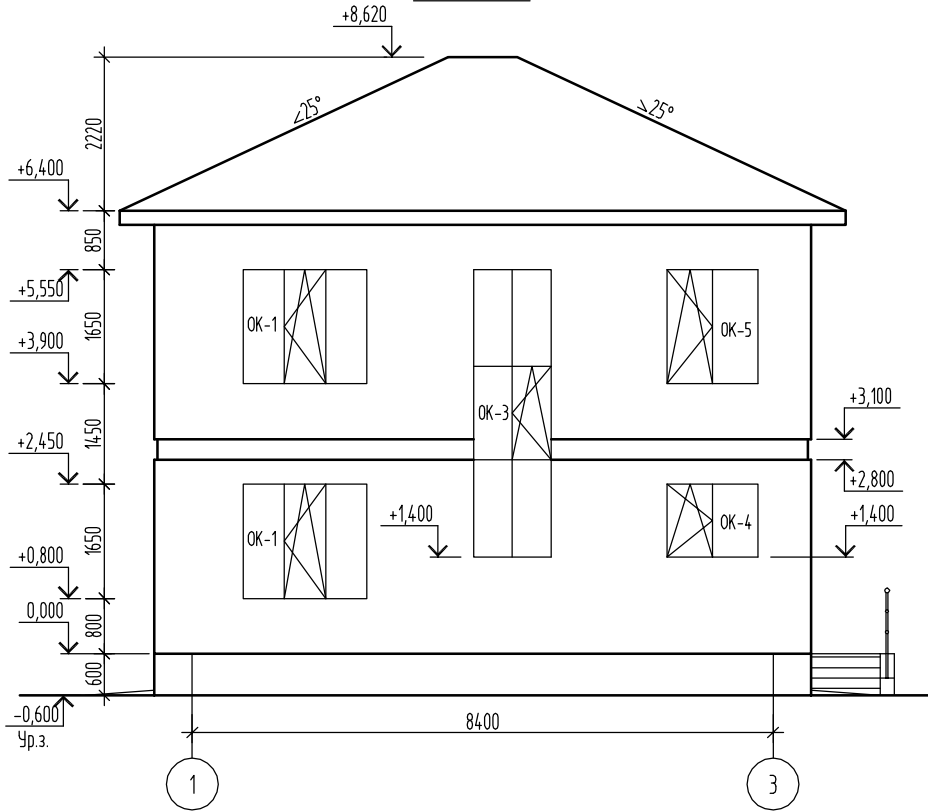
Фасад 1-3
