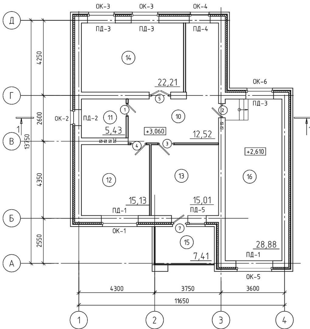
План 2 этажа
