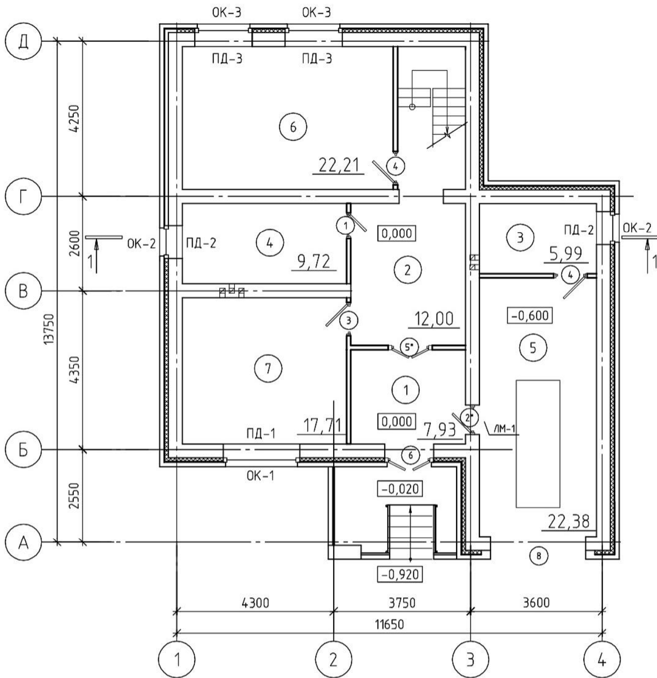
План 1 этажа
